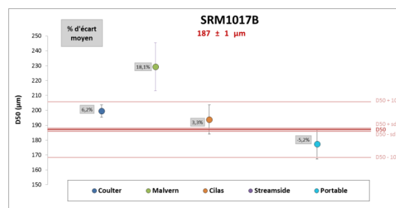
Figure 19 : Ecarts moyens des D50 \pm SD obtenus pour les granulomètres lasers BC LS 13320, Malvern Mastersizer 2000 ; Cilas et LISST Portable à partir du standard NIST SRM1017b au D50 de 187 \pm 1\mu\text{m} .
