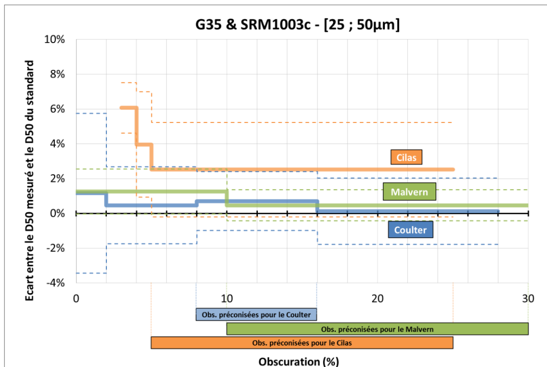
Figure 13 : Variation des écarts estimés entre la moyenne des D50 mesurés et la valeur des standards NIST-SRM1003c et G35, pour différentes gammes d'obscurités.
