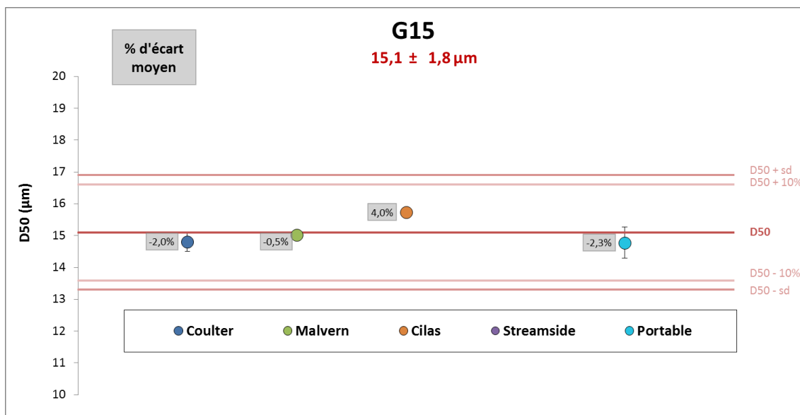
Figure 17 : Ecarts moyens des D50 \pm écart type (en \mu\text{m} ) obtenus pour les granulomètres lasers BC LS 13320, Malvern Mastersizer 2000 ; Cilas ; LISST Streamside et LISST Portable à partir du standard G15 au D50 de 15,1 \pm 1,8\mu\text{m} .
