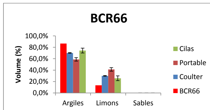
Figure 24 – Volume de chaque texture simple pour l’analyse du BCR66 par les trois appareils.
