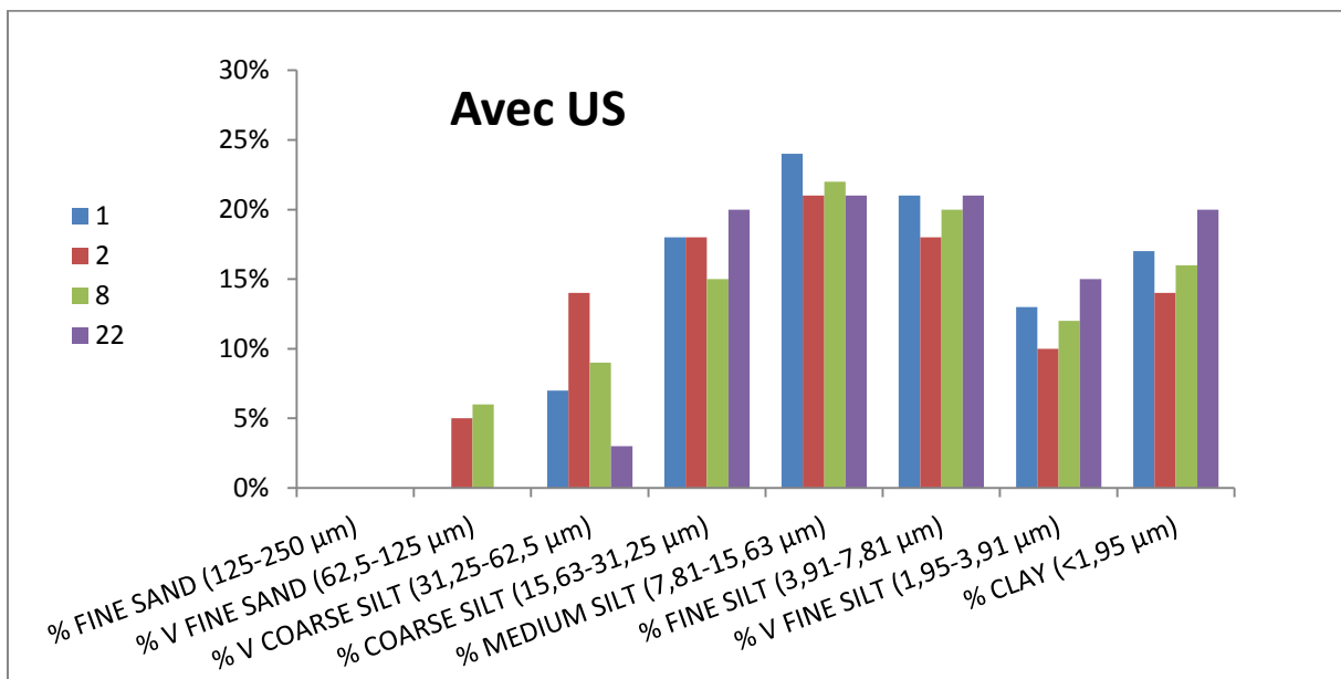
Figure 37 – Analyses de l'échantillon BAC-MAN-161122 avec utilisation des ultrasons sur le granulomètre Beckman Coulter après 1 ;2 ;8 et 22 jours de stockage.
