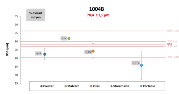
Figure 18 : Ecarts moyens des D50 \pm SD \pm 10% obtenus pour les granulomètres lasers BC LS 13320, Malvern Mastersizer 2000 ; Cilas ; LISST Streamside et LISST Portable à partir du standard NIST SRM1004b au D50 de 71 \pm 1,8\mu\text{m} .
