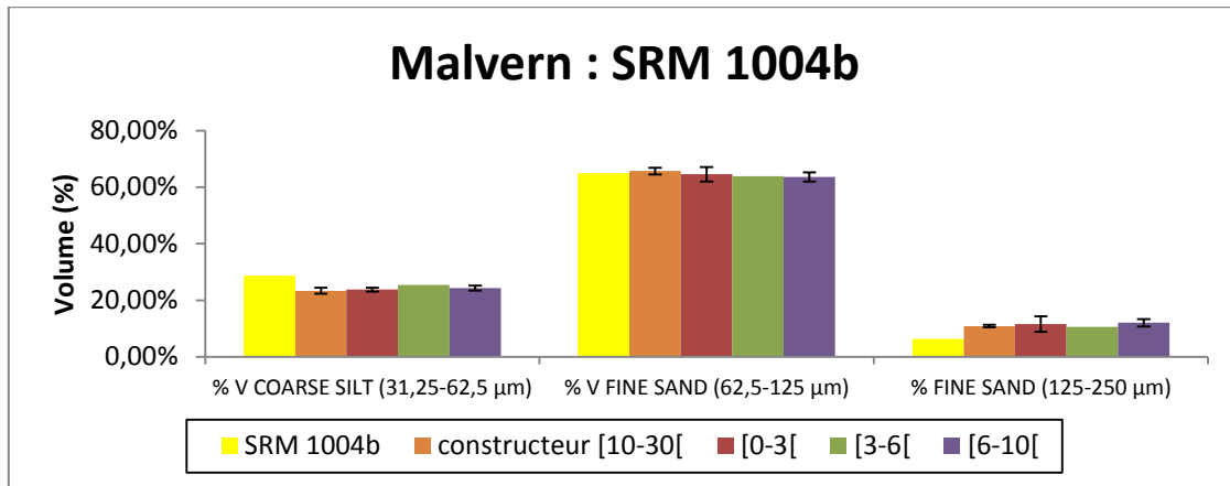
Figure 15 - Distribution granulométrique des textures détaillées en fonction des gammes d'obscurisation ([0-3[% ; [3-6[% ; [6-10[%; constructeur [10-30[%) pour le granulomètre Malvern à partir du standard certifié NIST SRM 1004b.
