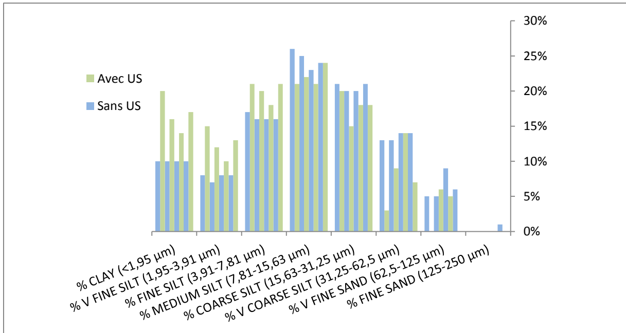
Figure 39 – Comparaison des analyses de l'échantillon BAC-MAN-161122 avec et sans utilisation des ultrasons sur le granulomètre Beckman Coulter après 1, 2, 8 et 22 jours de stockage.
