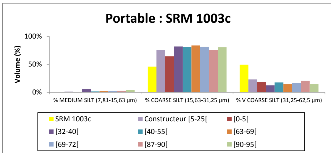
Figure 16 - Distribution granulométrique en fonction des gammes de transmissions ([0-5% ; [5-27% ; [32-40% ; [40-55% ; [63-69% ; [69-72% ; [87-90% ; [90-95% ; constructeur [5-25]) pour le granulomètre LISST Portable (v1) à partir du standard certifié NIST SRM 1003c.
