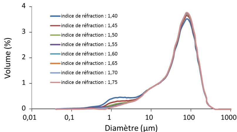
Figure 8 – Distributions granulométriques d'un même échantillon prélevé dans le Rhône à la station de Jons obtenues à partir d'indice de réfraction différents entre 1,4 et 1,75.
