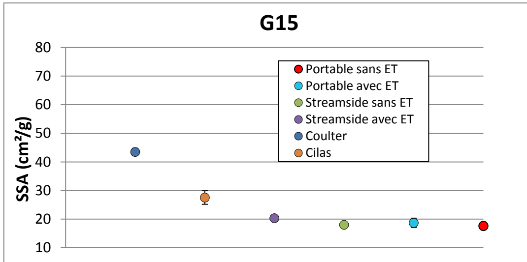
Figure 22 - Ecart moyen des SSA obtenus pour les granulomètres lasers Coulter ; Streamsides ; Portable (v1) et Cilas dans les gammes d'obscurations constructeurs à partir du standard G15 à la SSA de 37.9 cm 2 /g.
