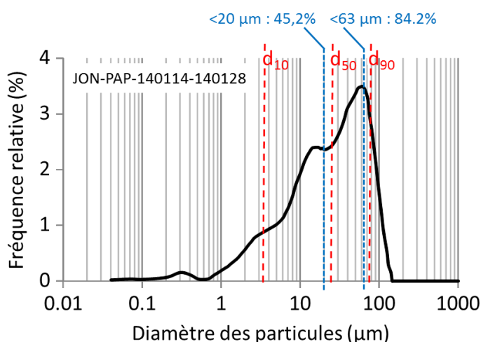
Figure 42 - Distribution granulométrique d'un échantillon de MES prélevés à l'aide d'un PAP (du 14 au 28 janvier 2014) à Jons. Les indices de classement de Trask (2,3) et d'asymétrie (0,8) sont typiques des indices calculés pour les échantillons de MES prélevés à Jons par centrifugation ou à l'aide de PAP.
