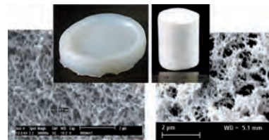
Exemple de matrices cellullosiques issues du projet NANOCEL : acétate de cellulose réticulé (gauche) et aérocellulose (droite)
