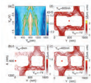
Mise en évidence théorique d'un paradoxe de Braess quantique dans un stade rectangulaire cohérent. La fermeture du bras médian par effet de grille (de (b) à (d)) se traduit paradoxalement par une augmentation de la conductance totale du dispositif (a). La microscopie SGM permet de confirmer expérimentalement l'effet. D'après M.G. Pala et al. (à paraître).
