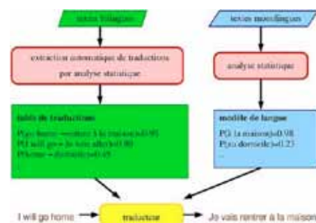
Principe de la traduction automatique statistique.
