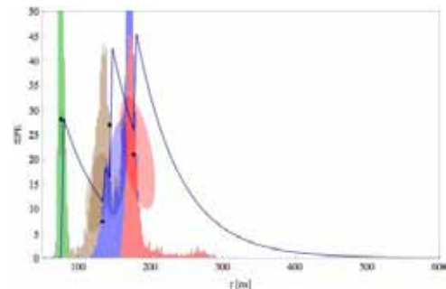
Inférence par simulation dans l'expérience Pierre Auger.
