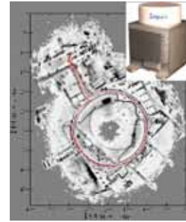
Associé à des algorithmes de SLAM, le Radar permet à un véhicule de se localiser tout en construisant au cours du déplacement une carte de son environnement.
