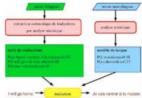
Principe de la traduction automatique statistique.
