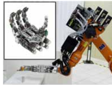
Plateforme robotique dédiée à la manipulation dextre et modèle CAO de la main ABILIS.
