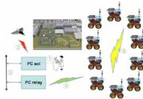
Architecture du projet R-Discover avec un drone et une flotte de robots terrestres.
