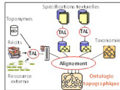
Approche générale suivie pour la constitution de l'ontologie topographique.
