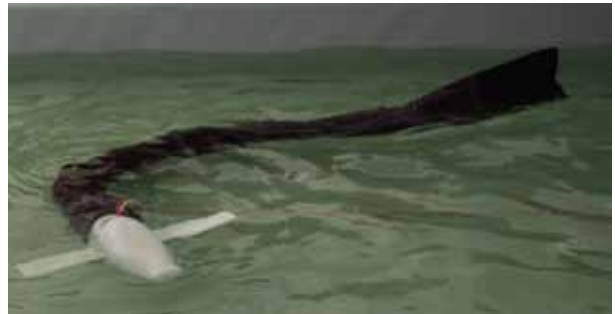
Robot RAAMO en action durant le workshop Bio-inspired robot 2011, Nantes 6-8 Avril 2011.
