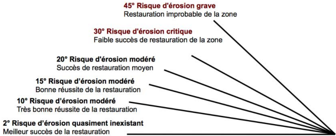
Figure 17 : Influence de la pente sur l'érosion et le succès de la revégétalisation. Epandage d'un substrat minimum de 30cm ne nécessitant pas de moyens de stabilisation possible jusqu'à 20°. Au delà et jusqu'à 30°, il devient nécessaire de mettre en place des dispositifs de stabilisation des ouvrages restaurés, de plus en plus importants. Au delà de 30°, les surfaces à restaurer ne permettent plus de retenir les épaisseurs de 30 cm de substrat, compromettant le développement d'un couvert végétal et la pérennité de la zone restaurée.
