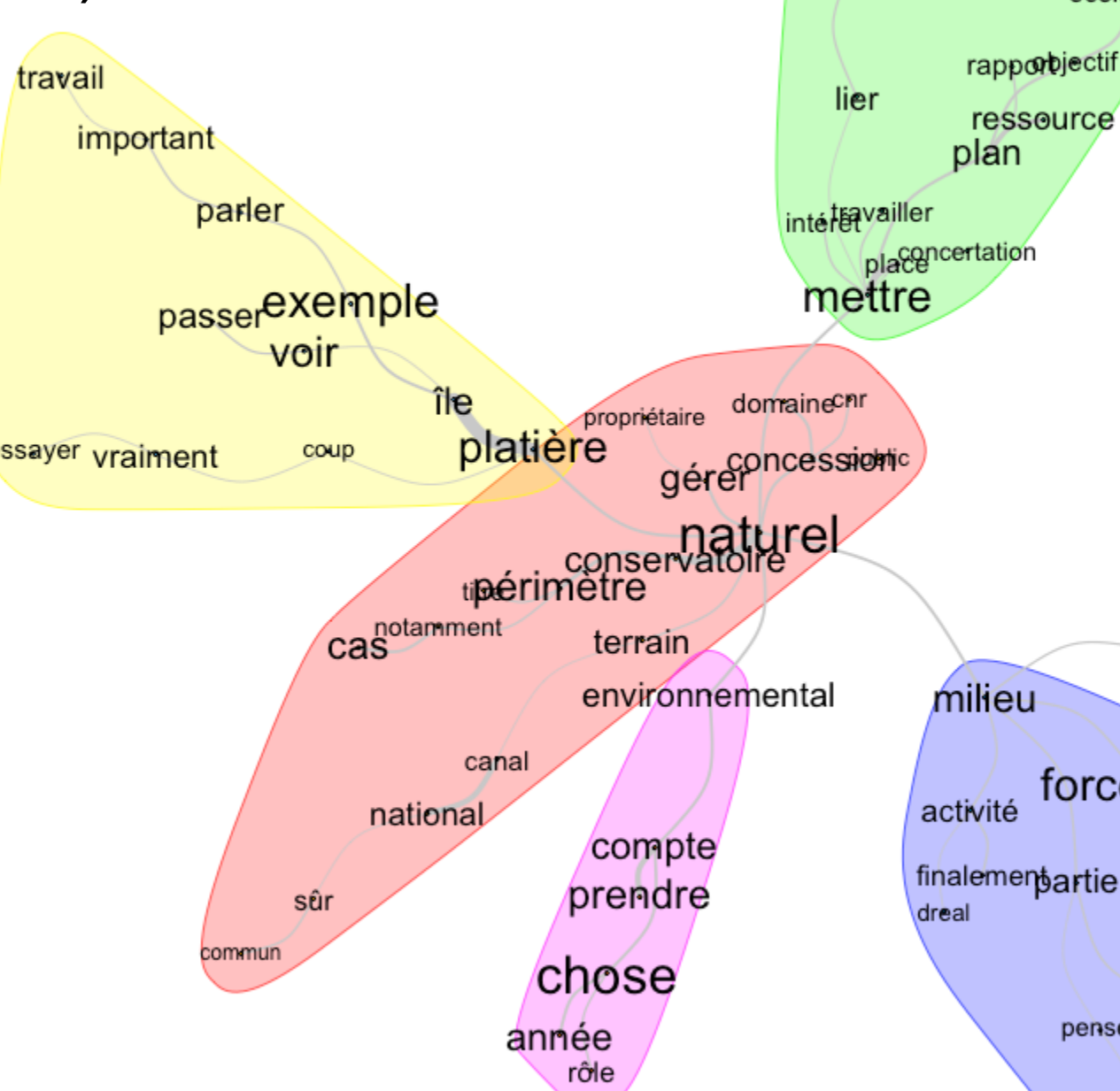
Fig. 6. Graphes des similitudes réalisés sous IRaMuTeQ - Des discours centrés sur des territoires de nature où les acteurs sont en tension pour concilier différents enjeux. A) Miribel : électricité, navigation, ressource en eau, biodiversité, demande foncière, granulats, fréquentation) ; B) Platière : pollution de l'air, partage de la ressource, gestion foncière et forestière.
