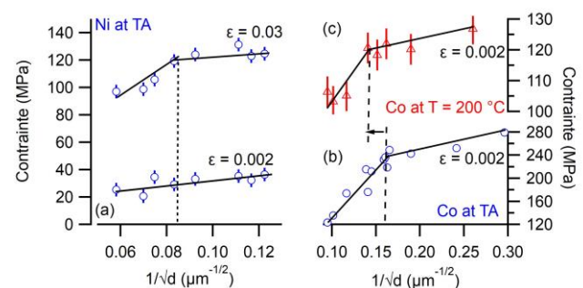
Figure 1. Loi de Hall-Petch à température ambiante pour le nickel à deux niveaux de déformation (a). Loi de Hall-Petch pour le cobalt pour une de déformation totale de 0,002 à température ambiante (b) et 200 °C (c).
