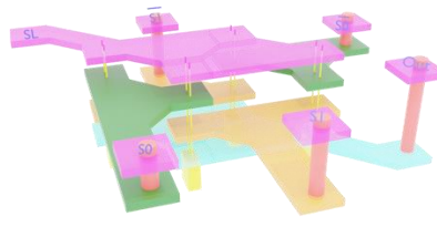
Fig. 17. 2-input non-volatile LUT.
