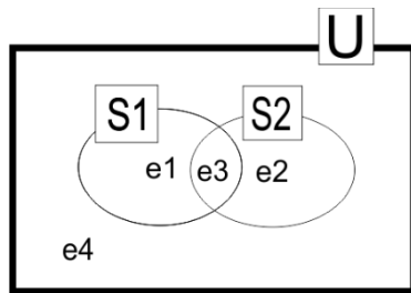
Fig. 2. Euler-Venn diagram
