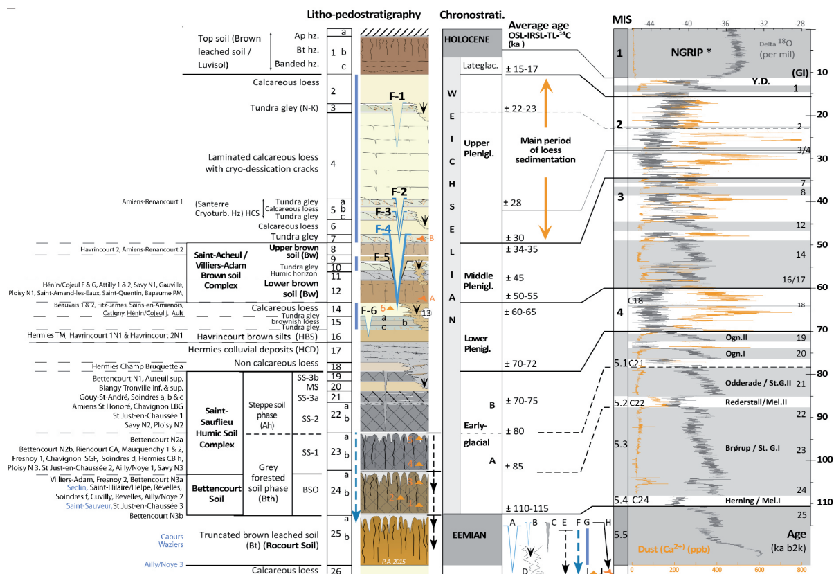
Fig. 5 - Cadre chronostratigraphique du Weichselien et position des différents sites paléolithiques : état des connaissances actuelles (d'après ANTOINE et al. 2016 et ANTOINE & LOCHT 2015, modifié).
