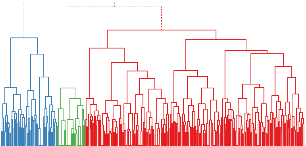
Dendrogramme (3 groupes)
