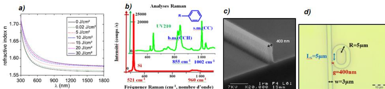
Figures - a) Ellipsométrie de l'UV210 à insulations variables b) Analyses et imageries Raman c,d) Microscopies (électronique à balayage et optique) pour structures photoniques intégrées
