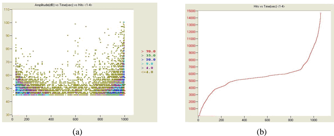
FIG.4 – Evolution de l'activité acoustique au cours d'un essai de fluage : a) Amplitude ; b) nombre de signaux cumulés.
