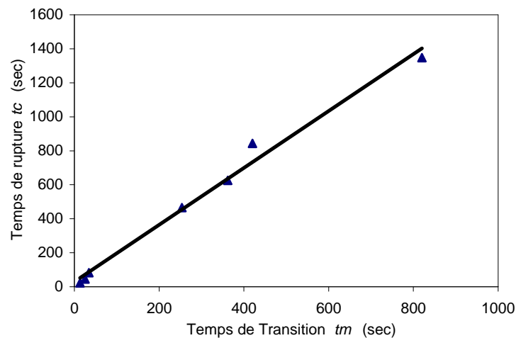
FIG.8 – Corrélation entre la durée du fluage primaire t_m et le temps à rupture t_c .
