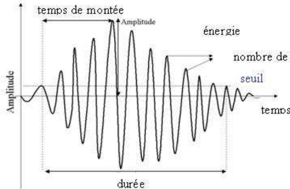
FIG.3 – Principaux paramètres mesurés sur une salve d'émission acoustique
