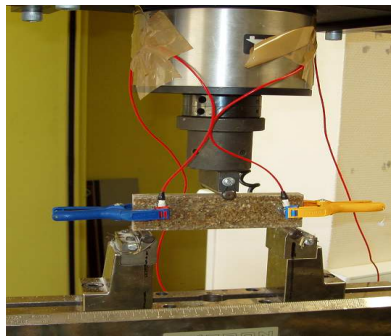
FIG.1 – Essai de fluage en flexion 3-points sur des éprouvettes en béton à base polymère
