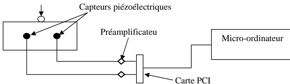
FIG.2 – Synoptique d'un système d'émission acoustique.
