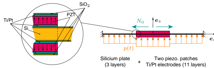
FIG. 5 – Schéma du système
