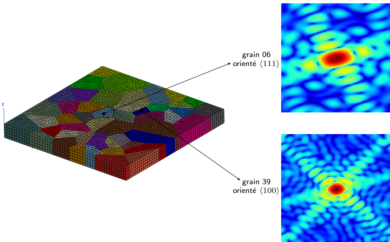
FIG. 2 – Illustration de la méthodologie de calcul : maillage du film polycristallin et exemple de calcul de taches de diffraction en l'absence de déformation (seule la forme des grains joue).
