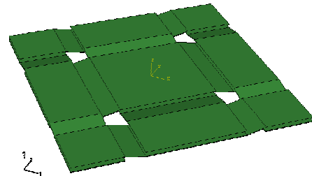
FIG. 4 - Model mésoscopique de taffetas pour l'étude méso/macro (216 DDLs)
