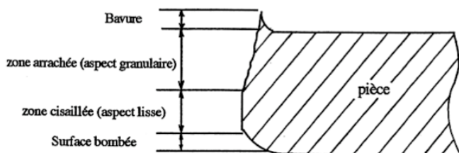
FIG. 3 : Longueurs caractéristiques du bord découpé [3]
