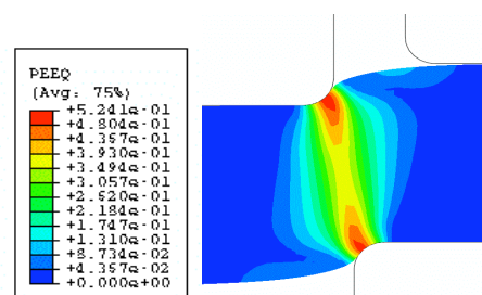
FIG. 6 : Contour de déformations plastiques équivalentes (23% de pénétration)
