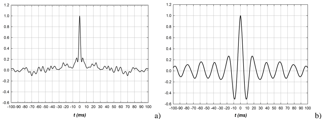
Figure 6: a) Coefficient d'autocorrélation du taux d'entraînement du jet marguerite à X=3D_e ; b) Coefficient d'autocorrélation du diamètre D_{TD} du jet marguerite à X=3D_e .
