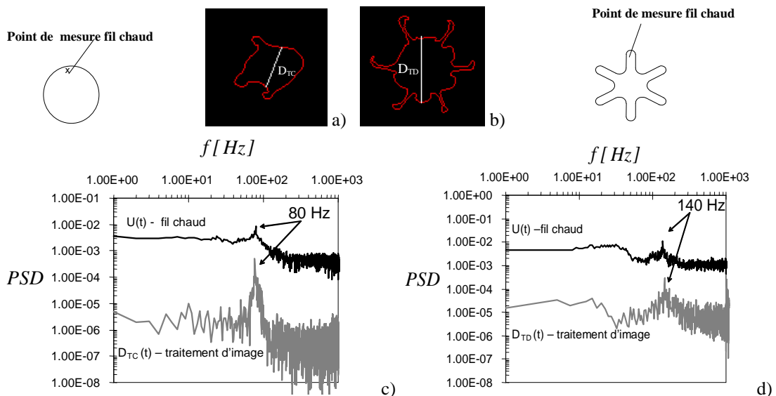
Figure 3: Contours des images à X=1D_e : a) Jet circulaire, b) Jet marguerite; Comparaison des spectres de la vitesse et de la dimension du jet: c) Jet circulaire, d) Jet marguerite
