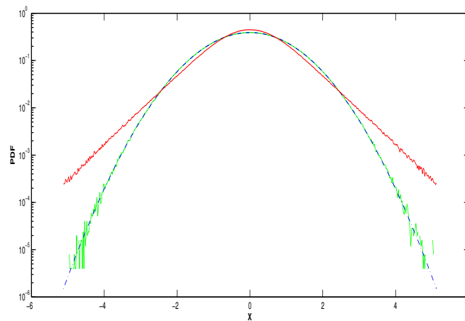
FIG. 3 – Fonction de densité de probabilité des pentes des surfaces simulées à partir du modèle hydrodynamique. Ligne bleue pointillée : Loi Gaussienne. En vert : loi de probabilité des surfaces linéaires. En rouge : Loi de probabilité des surfaces nonlinéaires
