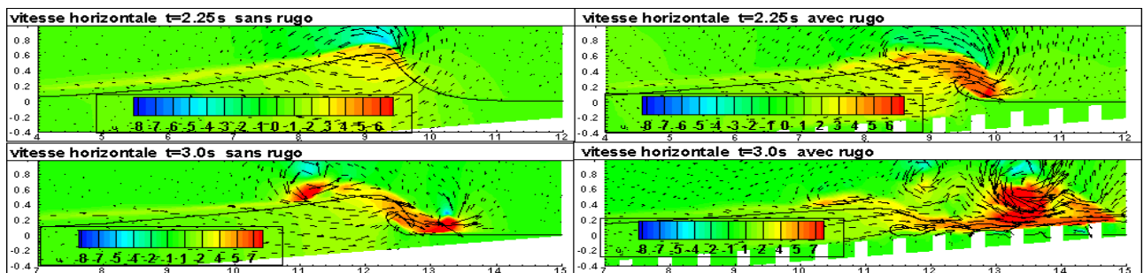
FIG.9 .Vitesses horizontales à t=2.25s et 3.s , pour le cas « ruغو » (droite) et « non-ruغو » (gauche).
