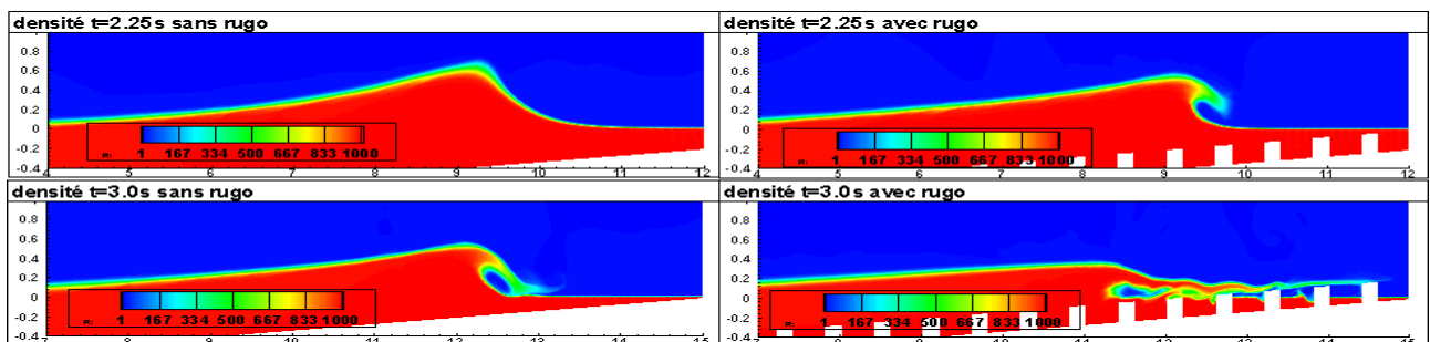
FIG.10 .Densité à t=2.25s et 3.s , pour le cas « ruغو » (droite) et « non-ruغو » (gauche).
