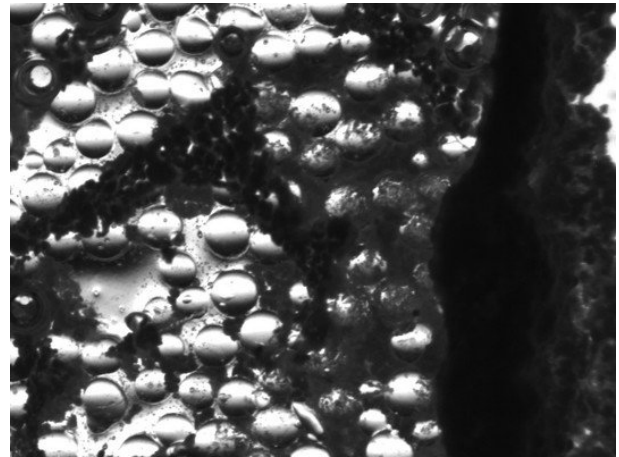
FIG. 7 – Large croûte de sulfate de sodium formée à la surface (la taille des grains est 500 \mu m).
