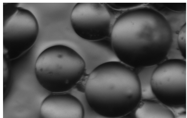
FIG. 5 – Cristaux de halite précipités au contact entre les billes (la taille des grains est 500 \mu m).
