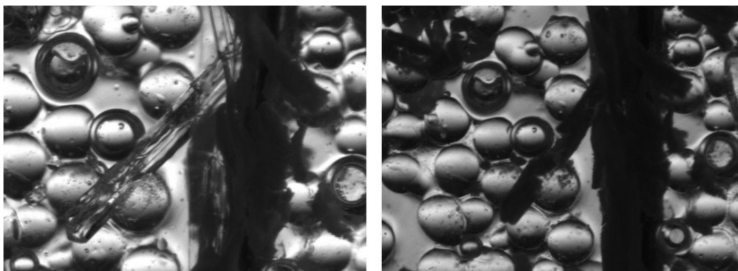
FIG. 8 – Déshydratation d'un cristal de mirabilite en thénardite entre 20 et 80h de séchage. Les nombreux cristaux de thénardite obtenus gardent la forme du cristal initial de mirabilite (la taille des grains est 500 \mu m).
