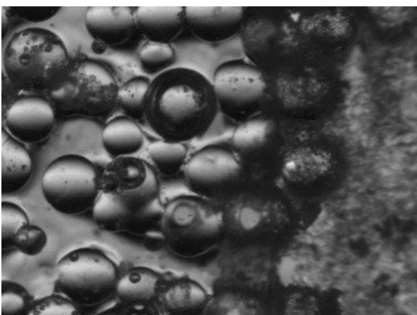
FIG. 4 – Fine croûte de chlorure de sodium formée à la surface (la taille des grains est 500 \mu m).
