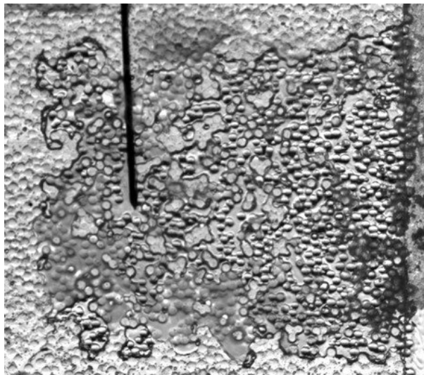
FIG. 3 – Réseau poreux modèle imprégné entièrement de solution saturée de chlorure de sodium après 20h de séchage à température ambiante (la taille des grains est 500 \mu m).
