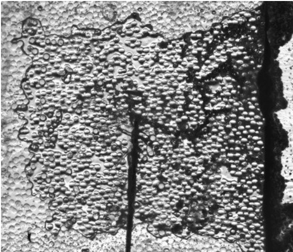
FIG. 6 – Réseau poreux modèle imprégné entièrement de solution saturée de sulfate de sodium après 20h de séchage à température ambiante (la taille des grains est 500 \mu m).
