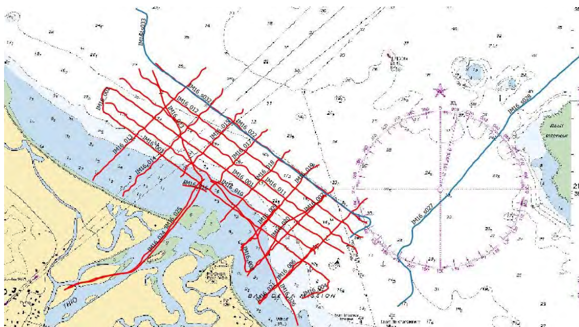
Figure 3. Plan de navigation du levé THR réalisé à l'embouchure de la rivière Thio (en rouge les profils boomer, en bleu les profils sparker).
