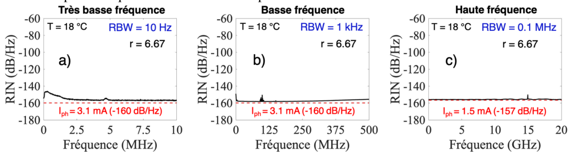
Fig. 2 : Spectres de RIN du laser EP-VECSEL. a) et b) RIN à très basse et à basse fréquence. c) RIN à haute fréquence. RBW : résolution de bande passante de l'analyseur de spectre électrique, r : taux de pompage. Les traits en pointillés rouges représentent le bruit de grenaille.
