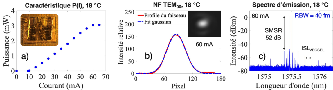
Fig. 1 : a) Caractéristique courant-puissance. b) Champ proche (NF) du mode transverse fondamental TEM_{00} . c) Spectre d'émission du laser en régime mono-fréquence. ISL : Intervalle spectral libre, RBW : résolution de bande passante de l'analyseur de spectre optique.
