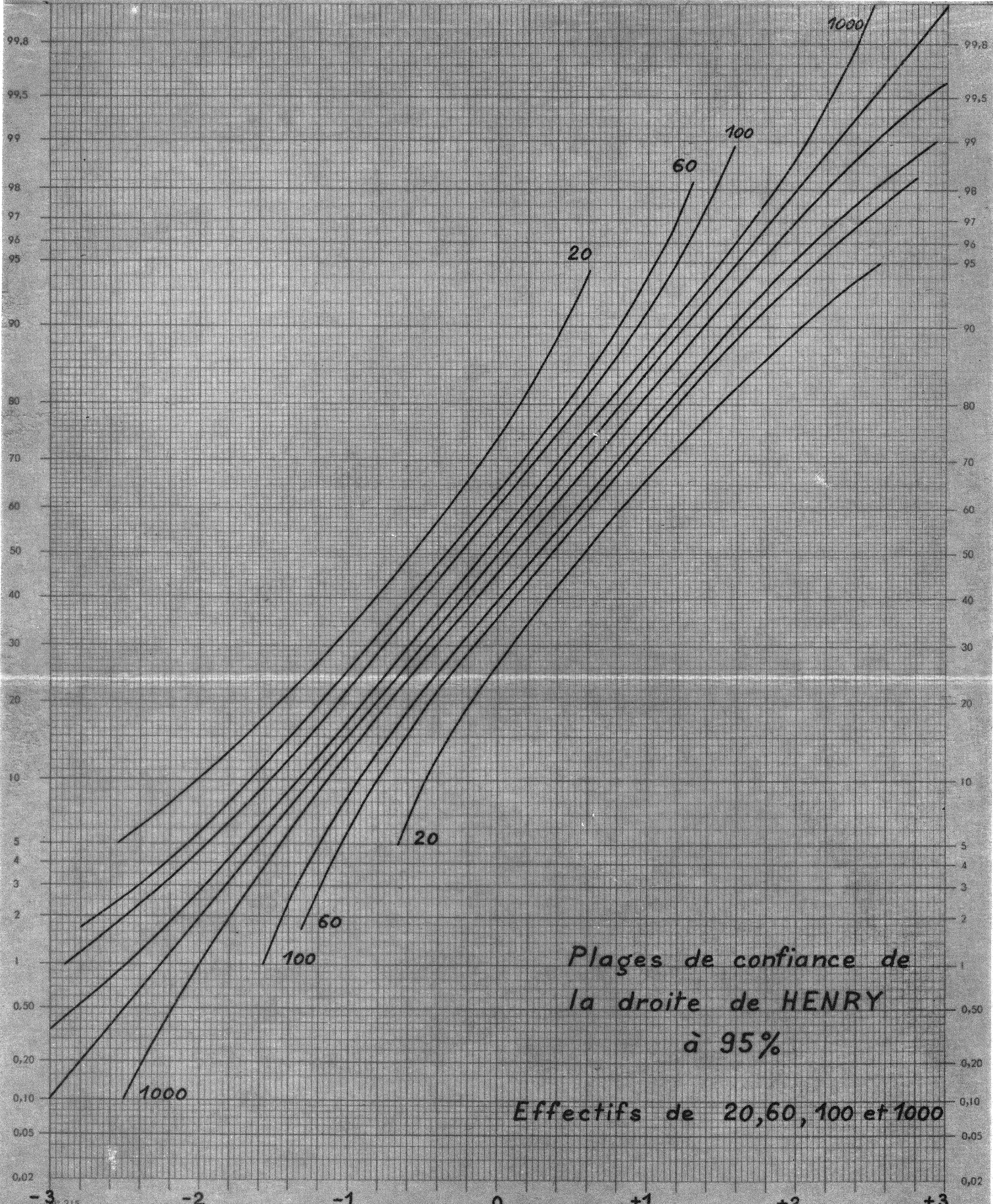
Diagramme de la droite de Henry ou droite-échantillon (anomorphe de la courbe de probabilité totale de la loi de Gauss).
