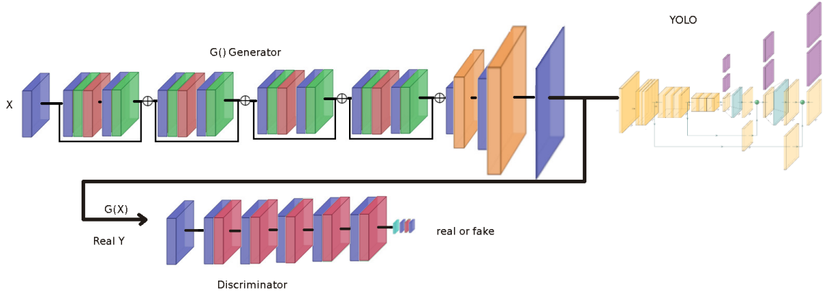
FIGURE 8 – Architecture SR WGAN avec l’ajout du réseau YOLOv3 comme réseau auxiliaire.
