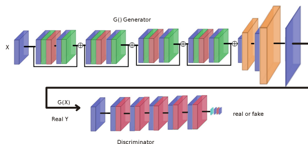
FIGURE 5 – Architecture de SR-WGAN avec en haut le générateur (réseau de super-résolution) et en bas le discriminateur. Les couches sont de type : convolution (bleu), réduction 1 \times 1 (bleu clair), activation ReLU (rouge), normalisation (vert), réarrangement (orange).
