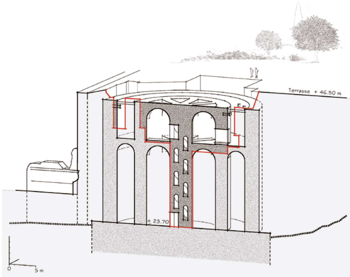
Fig. 9. Coupe mettant en évidence la position du soubassement de la cenatio rotunda au sein de la terrasse flavienne (dessin N. André, AMU-IRAA du CNRS).
