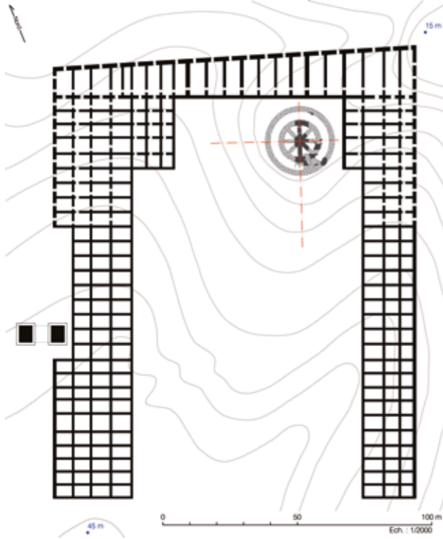
Fig. 10. Positionnement en plan de la cenatio rotunda au sein du terre-plein de la terrasse flavienne (dessin N. André, AMU-IRAA du CNRS).
