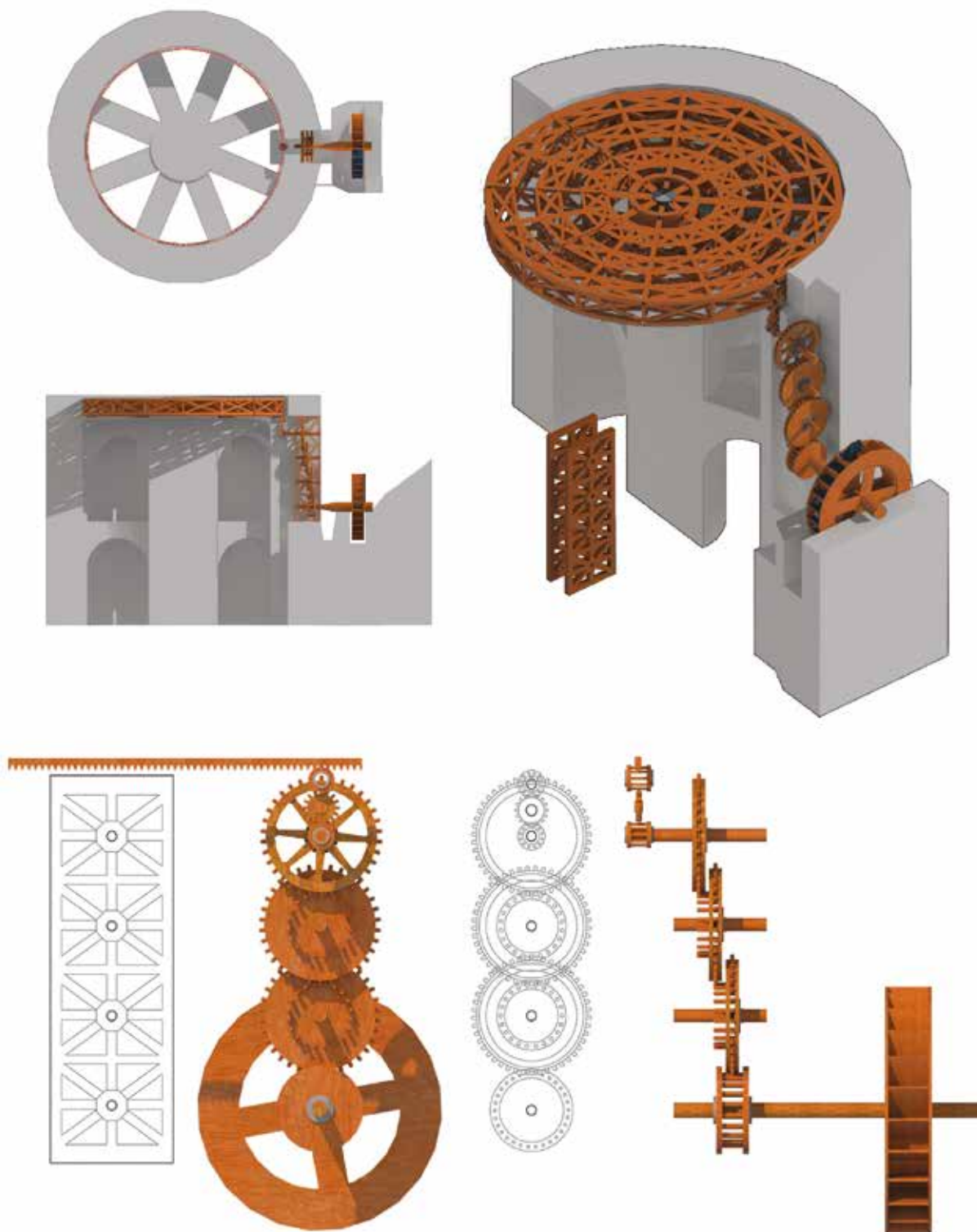
Fig. 5. Le mécanisme assurant la rotation du plancher mobile. Cette première hypothèse, élaborée et mise en forme par M. Gabay en 2013, devra être modifiée pour intégrer les résultats recueillis durant la campagne de 2014.
