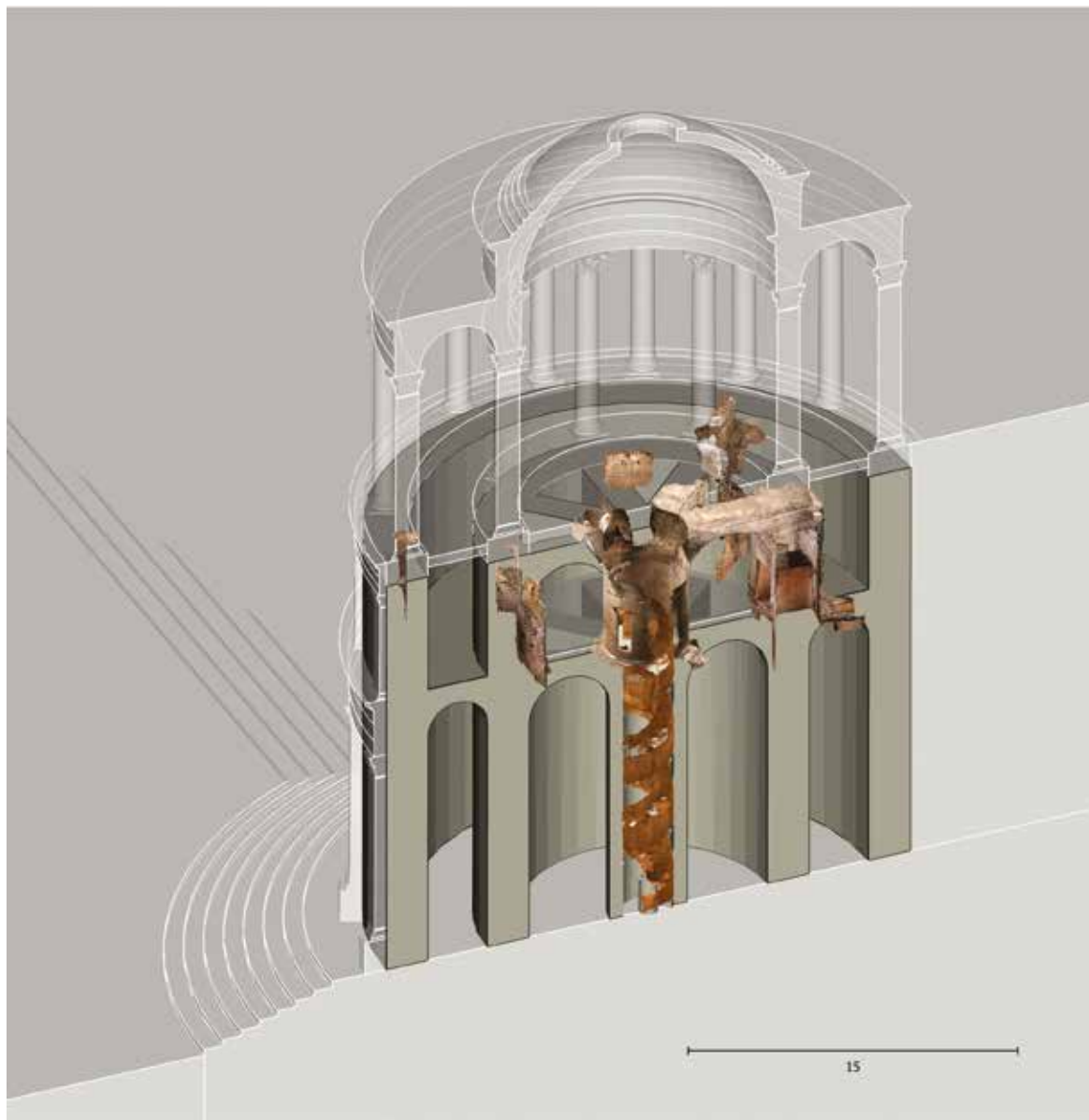
Fig. 6. Restitution de la cenatio rotunda élaborée à partir du relevé photogrammétrique. Les structures du soubassement dont l'existence et la forme sont dans la plupart des cas assurées apparaissent en gris foncé ; une trame plus claire et des contours blancs distinguent les parties et les détails dont la représentation repose uniquement sur des conjectures. La ligne horizontale tracée à droite, dans le prolongement du plancher tournant, suggère l'existence d'un corps de bâtiment lié à la "tour" et permettant un accès direct à la salle de banquet (dessin N. André, AMU-IRAA du CNRS).
