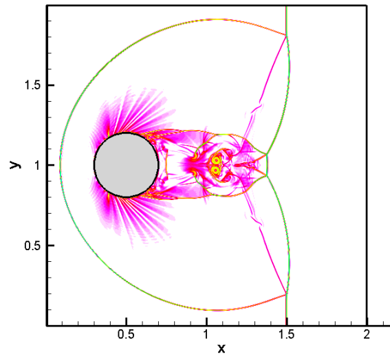
Figure 4 - Interaction d'un choc fort avec un cylindre de section circulaire à Re_D=5 \cdot 10^4 , obtenue à t=1,4 par un schéma OSMP7 et une technique de frontière immergée (1024×1024). Isovaleurs du module du gradient de masse volumique.
