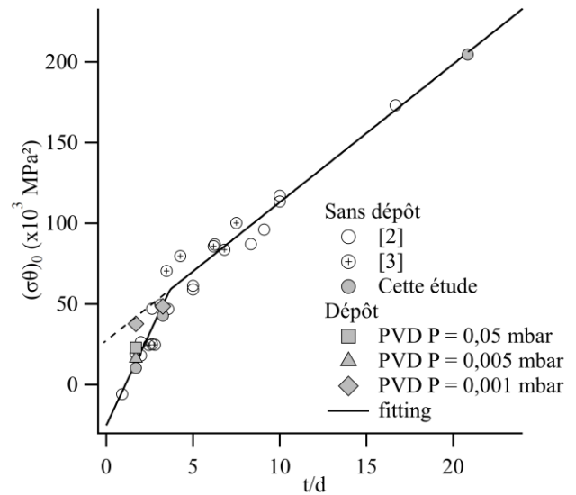
Figure 2. Evolution du paramètre (\sigma\theta)_0 , l'ordonnée à l'origine du stade II des courbes \sigma\theta = f(\sigma) , en fonction de du nombre de grains dans l'épaisseur pour des éprouvettes avec et sans dépôt
