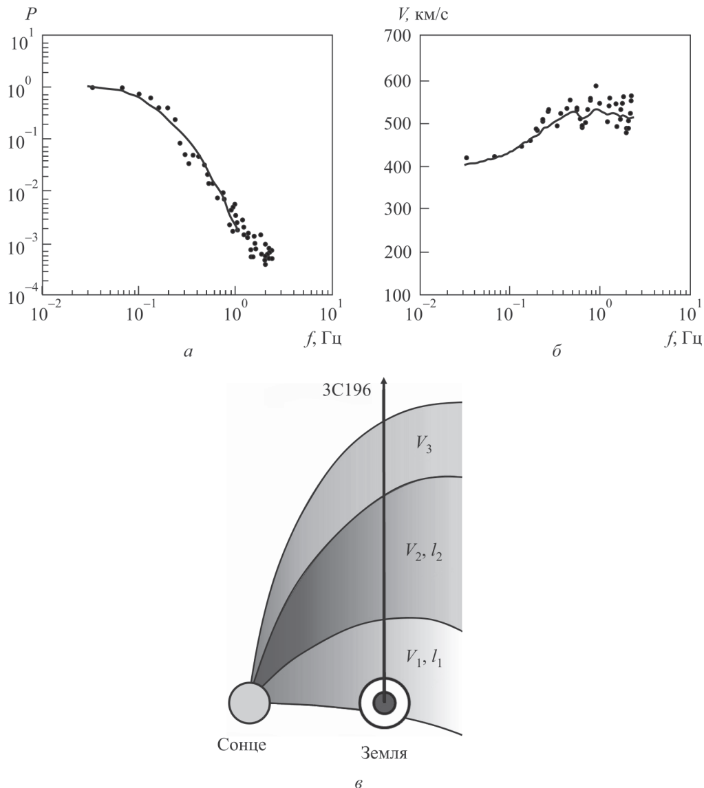
Рис. 8. Вписування теоретичних залежностей (суцільні лінії) в експериментальні дані (точки): a – спектри, б – дисперсійні залежності, в – реконструкція потокової структури сонячного вітру на промені зору на радіоджерело за сумісним аналізом спектра ( a ) та дисперсійної залежності ( б ). (Рисунок з роботи [52])
