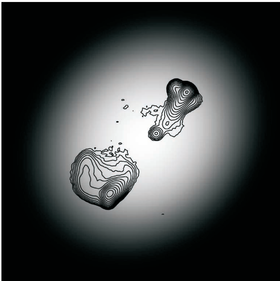
Рис. 45. Відкриття на декаметрових хвилях за допомогою РНДБ системи УРАН протяжних радіоструктур великої вибірки радіоґалактик і квазарів, які принципово відрізняються від радіозображень на високих частотах [14]
