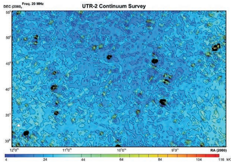
Рис. 44. Відкриття великої кількості дискретних та протяжних радіоджерел неперервного низькочастотного радіовипромінювання (емісійні туманності, залишки наднових, радіоґалактики, ґалактичний та позаґалактичний фон) [17]
