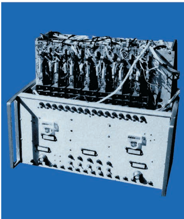
Рис. 32. Аналого-цифровий приймач для досліджень міжпланетних мерехтінгів та швидкоплинних процесів [14]
