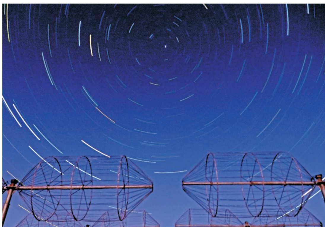
Рис. 69. Полярна зоря над антеною Північ–Південь радіотелескопа УТР-2 (час експозиції близько чотирьох годин)
