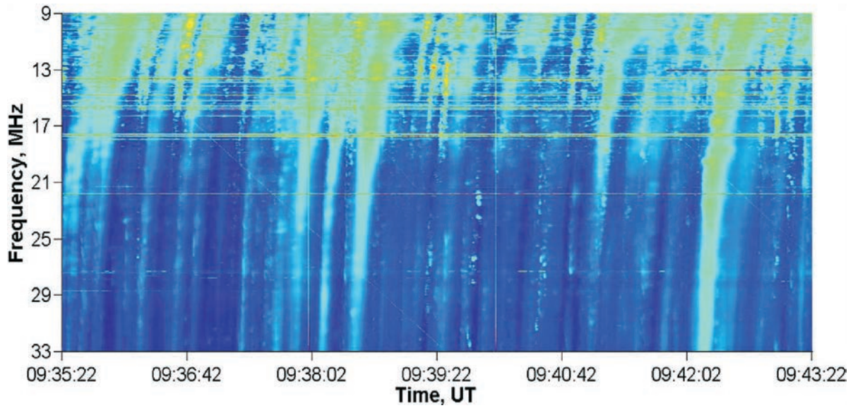
Рис. 39. Відкриття нових типів і особливостей спорадичного сонячного радіовипромінювання (спайки, сплески типу III-b та інші). Вдається реструктуризувати сонячну емісію навіть на частотах менших за 10 МГц, попри сильні радіозавади (горизонтальні лінії на динамічному спектрі) [17]
