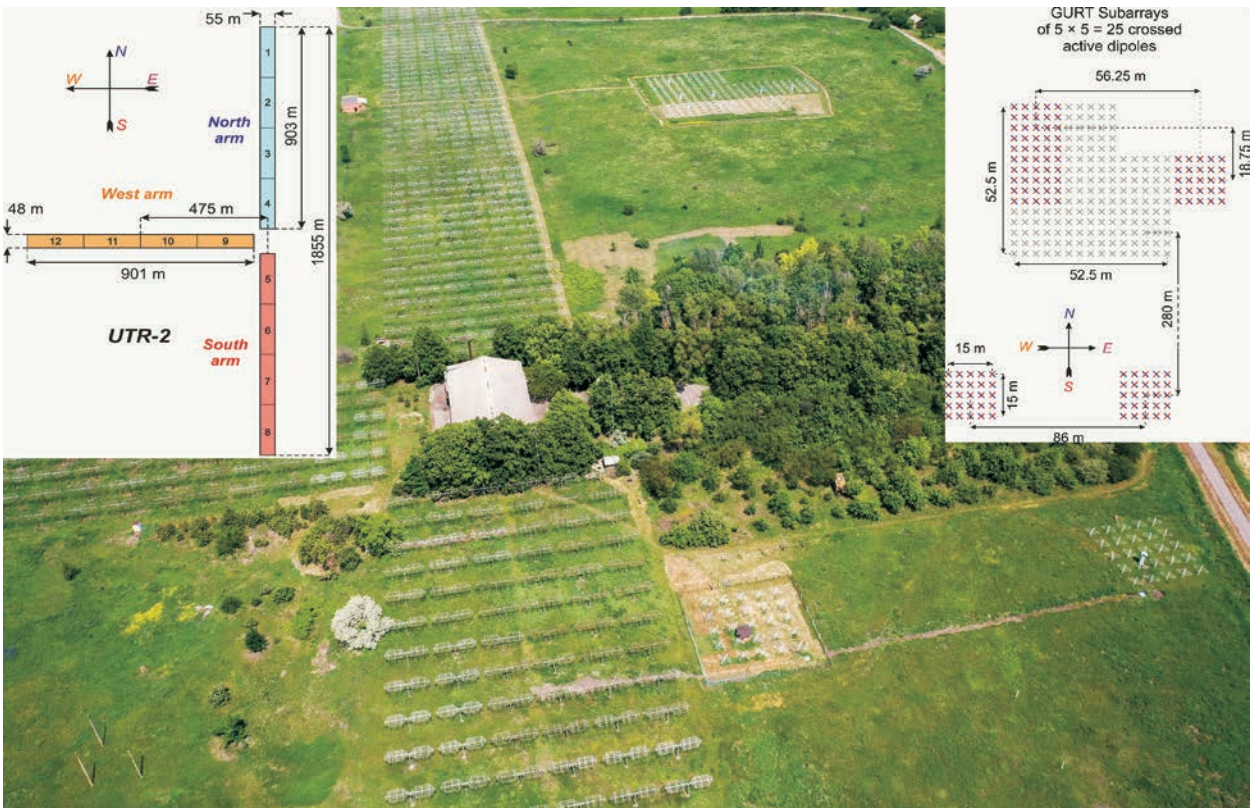
Рис. 27. Вигляд радіотелескопів УТР-2 та ГУРТ з висоти пташиного польоту
