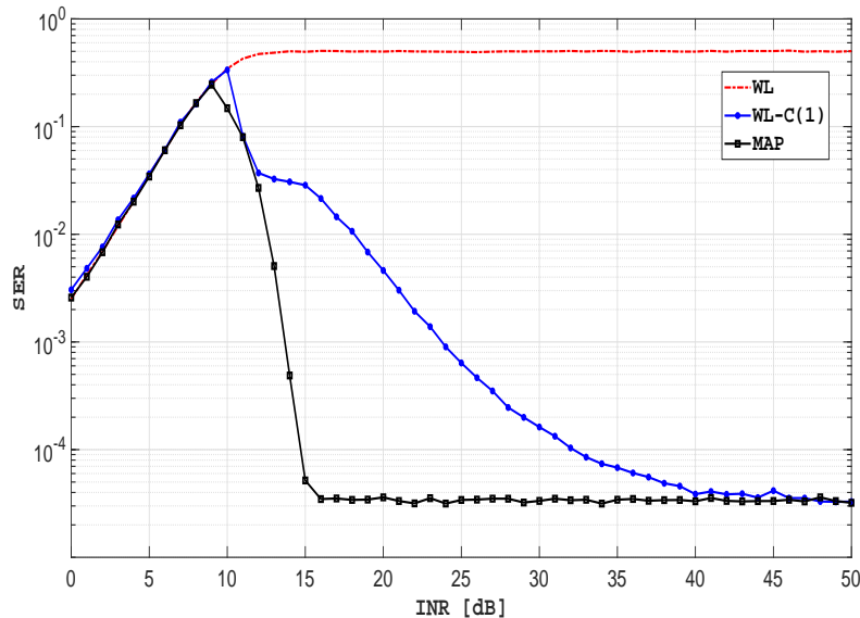
(a) SER
