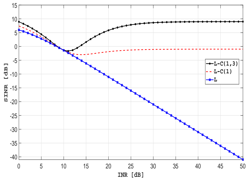
(b) SINR
