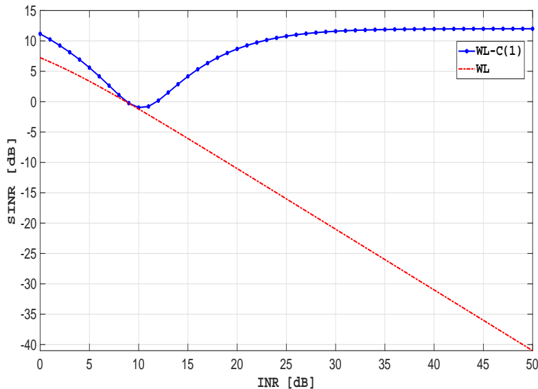
(b) SINR
