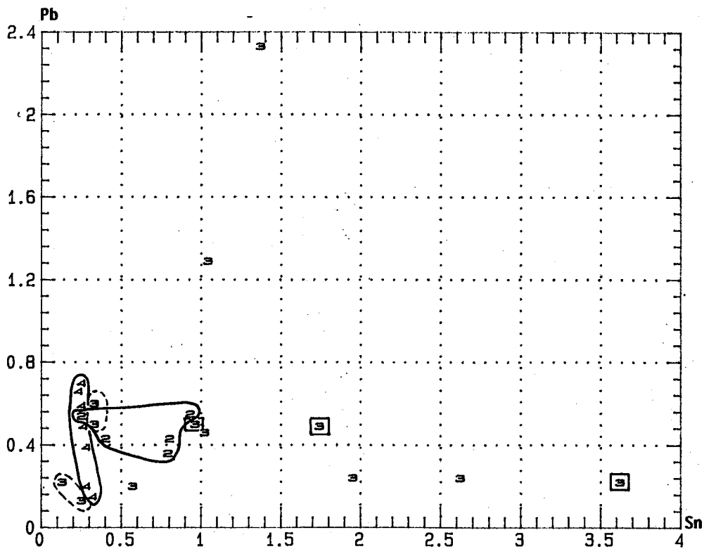
Schéma 6 - Types 2, 3 et 4 ; diagramme Pb/Sn \boxed{3} = fabricat raté ; \textcircled{3} = ressort type 3
