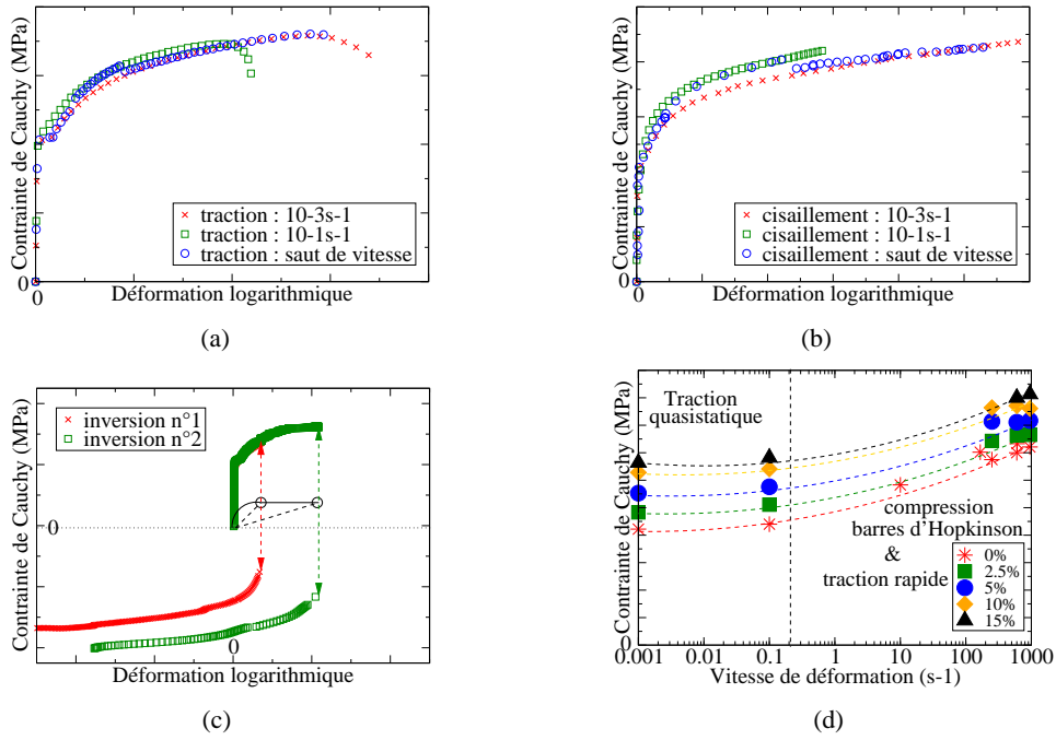
FIG. 2 – Résultats expérimentaux : (a) Traction axiale à 10^{-3} \text{ s}^{-1} et 10^{-1} \text{ s}^{-1} et saut de vitesse, (b) Cisaillement à 10^{-3} \text{ s}^{-1} et 10^{-1} \text{ s}^{-1} et saut de vitesse, (c) Cisaillement simple avec inversions de charge, (d) Traction axiale statique et dynamique et compression aux barres d’Hopkinson pour différentes valeurs de déformation plastique.
