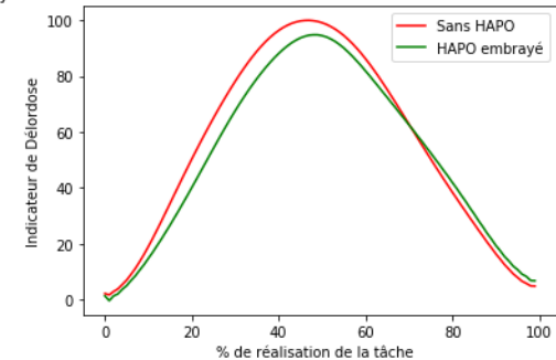
Figure 7: Courbe moyenne de l'indicateur de délordose lombaire Avec HAPO engagé et Sans HAPO (n=9).
