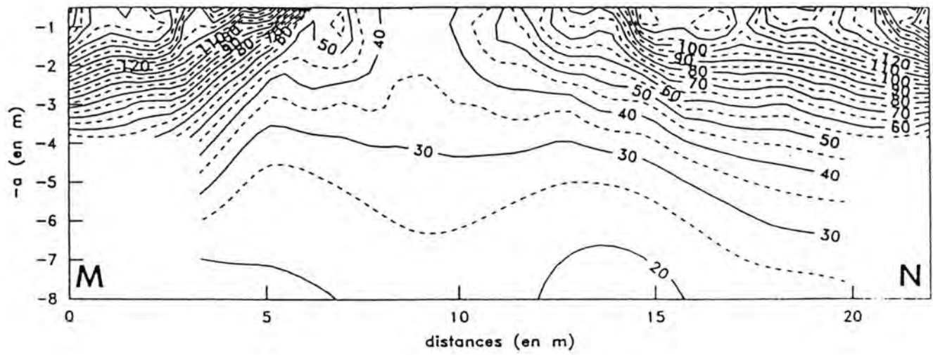
A B C PIECE D'EAU PS 1 Resistivite en (ohm.m)/ 10
