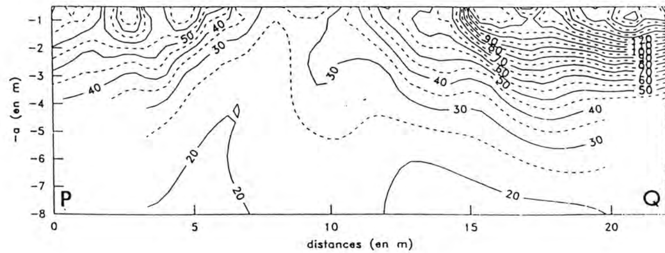
D E F G PIECE D'EAU PS 2 Resistivite en (ohm.m)/10
