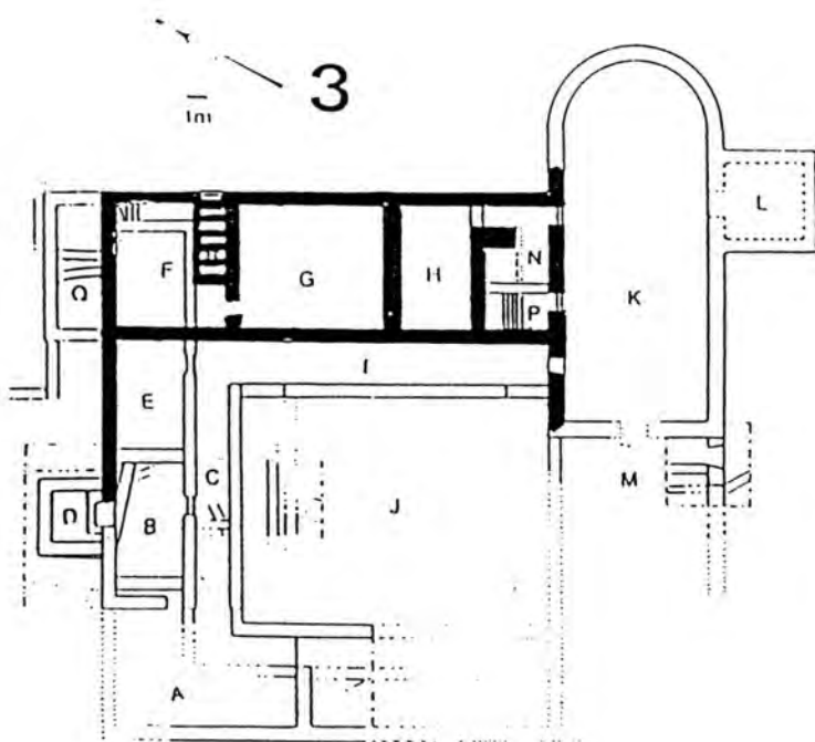
COUVENT DES CORDELIERS Principales phases de construction reconnues à la fouille (1993)
