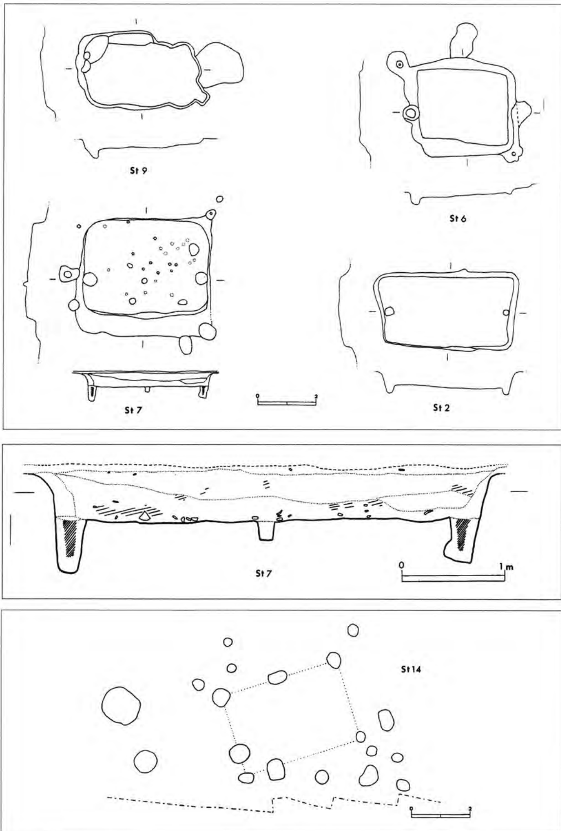
3. Plans et profils des fonds d'habitats excavés mis au jour en 1998.
