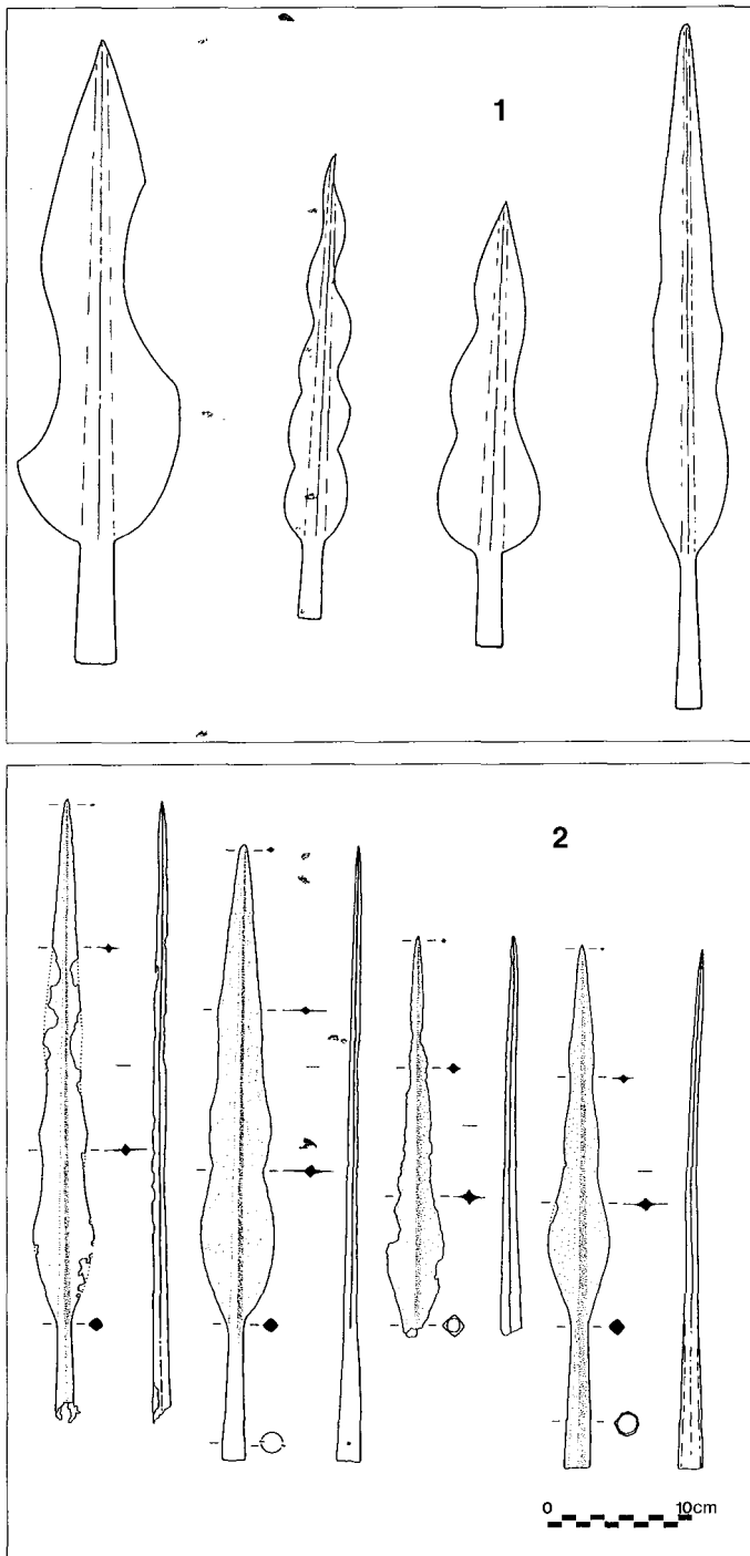
Fig. 3 - Les lances échan-crées type « Saône » et les autres types. 1. Les quatre types. 2. Quelques pointes de la Saône. Dessins C. Michel, musée Denon.
