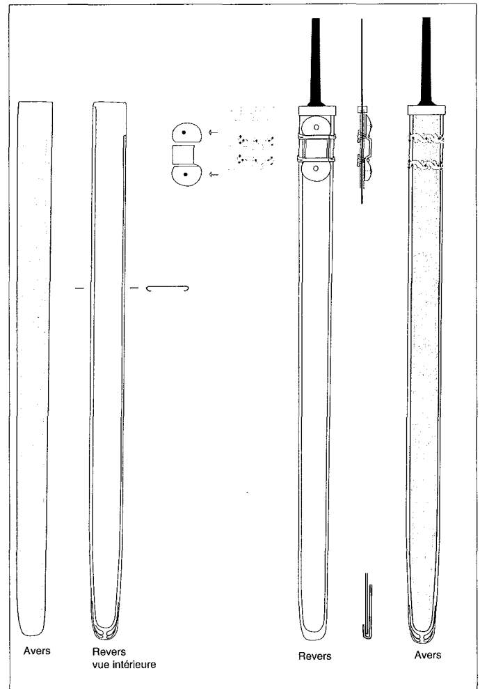
Fig. 2 - Le montage du fourreau de l'épée d'Allerey.
