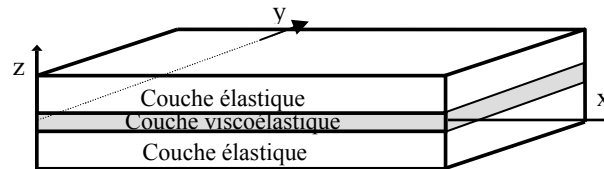
FIG. 1 - Tôle sandwich
