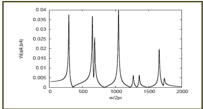
FIG. 4 - Courbe de réponse d'une plaque sandwich presque carrée : L=0.1778 , l=0.17 , excitation F(L/4, l/4)
