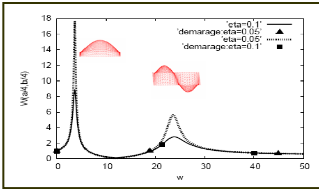
FIG. 3 - Courbes de réponses d'une plaque sandwich carrée en utilisant les approximants de Padé
