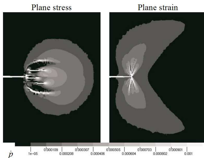
FIG. 4 – Vieillissement dynamique en pointe de fissure à 200 °C. Cartes des vitesses de déformation plastique ( \dot{\rho} )
