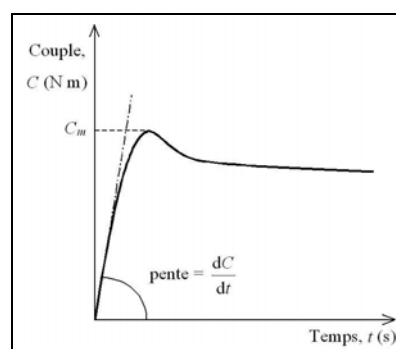
FIG. 1 – Evolution schématique du couple en fonction du temps.
