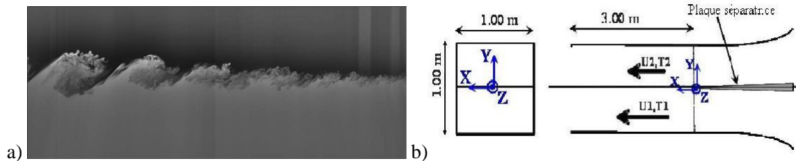
FIG. 3 – a) Visualisation de la couche de mélange par ensemençement de fumée dans la veine basse ( U_1 = 4\text{m/s} , U_2 = 2\text{m/s} , T_1 = 10^\circ , T_2 = 35^\circ ) ; b) Schéma de principe de l'écoulement de couche de mélange étudié dans la veine d'essai de la soufflerie.
