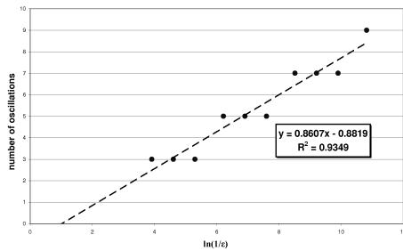
FIG. 12 – Nombre d'oscillations vs. \log(\varepsilon^{-1})
