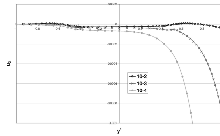
FIG. 13 – u_3 sur la ligne y^2 = 0 pour différents \varepsilon
