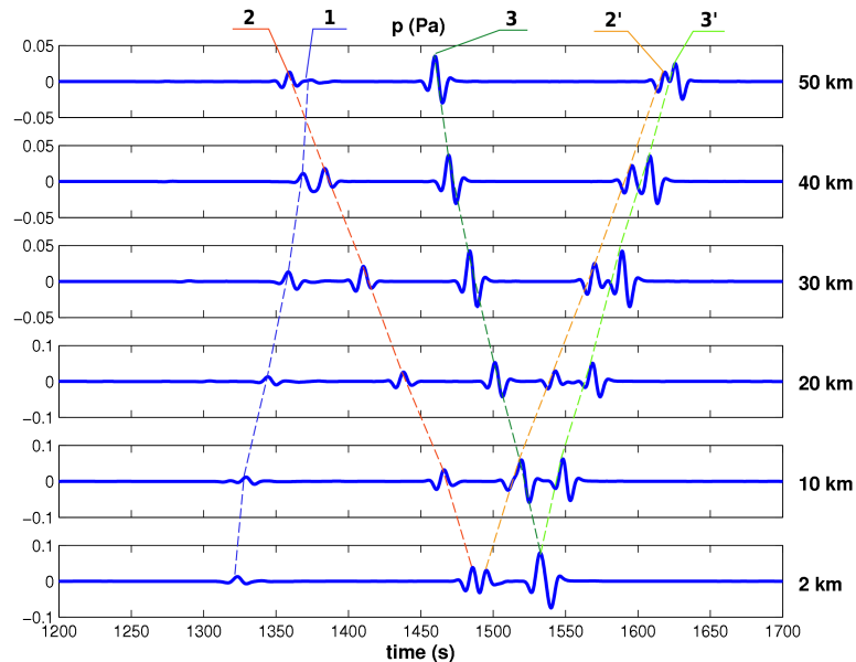
FIG. 3 – Signaux de pression en x = 400 km pour différentes altitudes ( \Delta = 300 m, CFL = 0.8 & \sigma_d = 0.01 ). 1 - ondes stratosphériques ; 2 - ondes thermosphériques réfractées entre 120 et 180 km d'altitude ; 2' - réflexion au sol des ondes thermosphériques 2 ; 3 - ondes thermosphériques réfractées à une altitude d'environ 115 km ; 3' - réflexion au sol des ondes thermosphériques 3.
