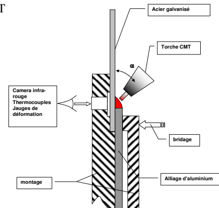
FIG. 2 – Dispositif expérimental
