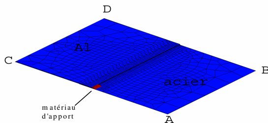
FIG. 7. Maillage utilisé (les plaques sont en bleu et le matériau d'apport en rouge)
