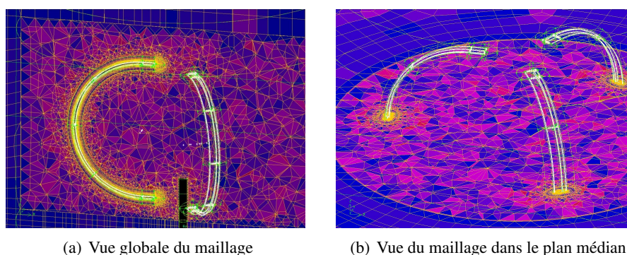
FIG. 4 – Éléments de maillage du domaine de calcul
