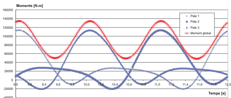
FIG. 8 – Moment global calculé
