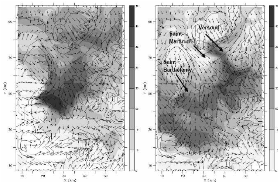
FIG. 2 – Concentration d'ozone due à la production locale pO_3 (en ppbV) et composante horizontale du champ de vent, à 15h les 5 aout (à gauche) et 6 aout (à droite)
